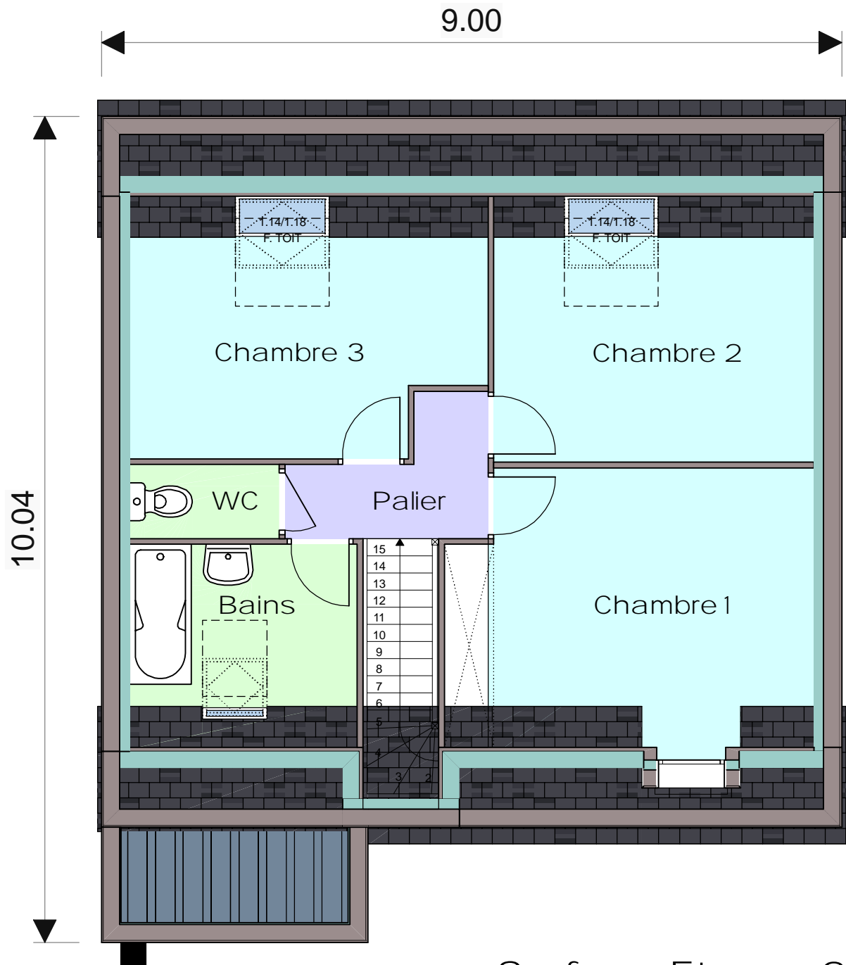
Surface Etage : 38.12 m 2
